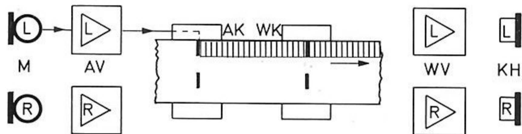
Synchron-Playback 1. Aufnahme
