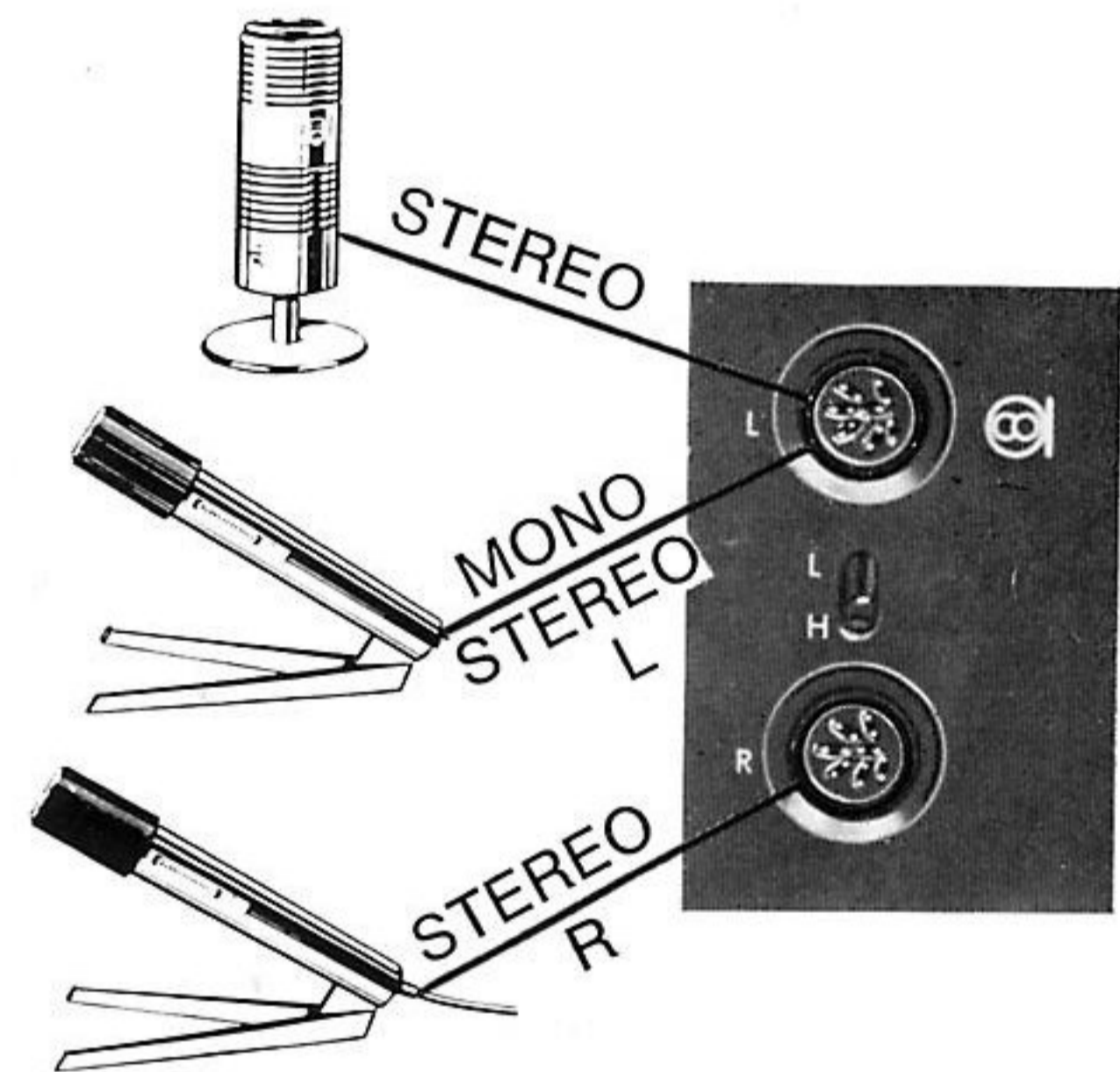
Mikrofonbuchsen
