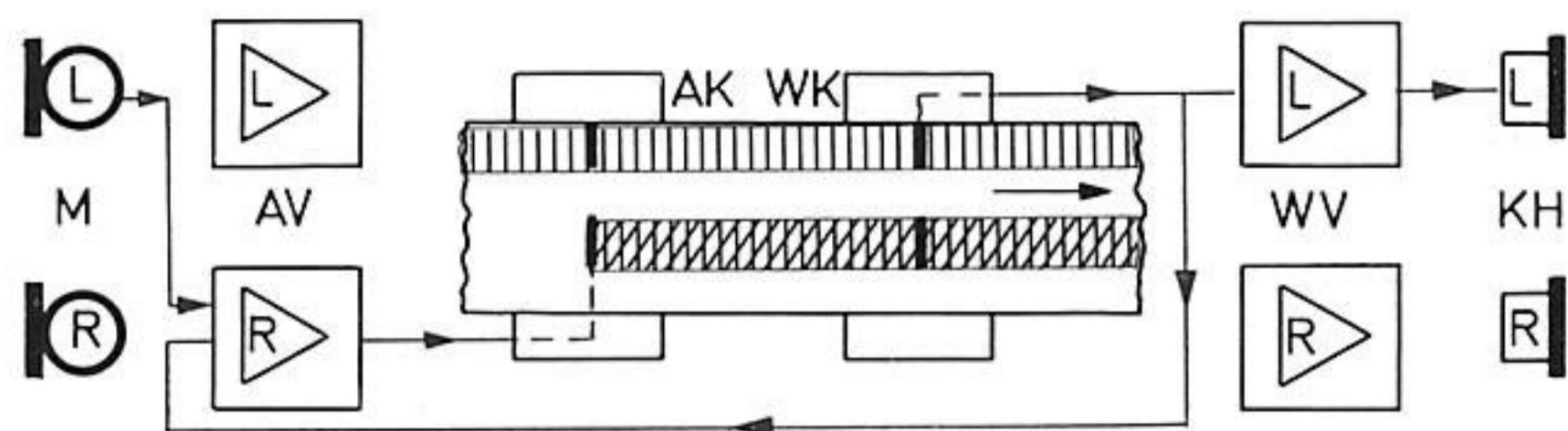
Multi-Playback 2. Aufnahme
