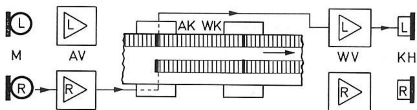
Synchron-Playback 2. Aufnahme
