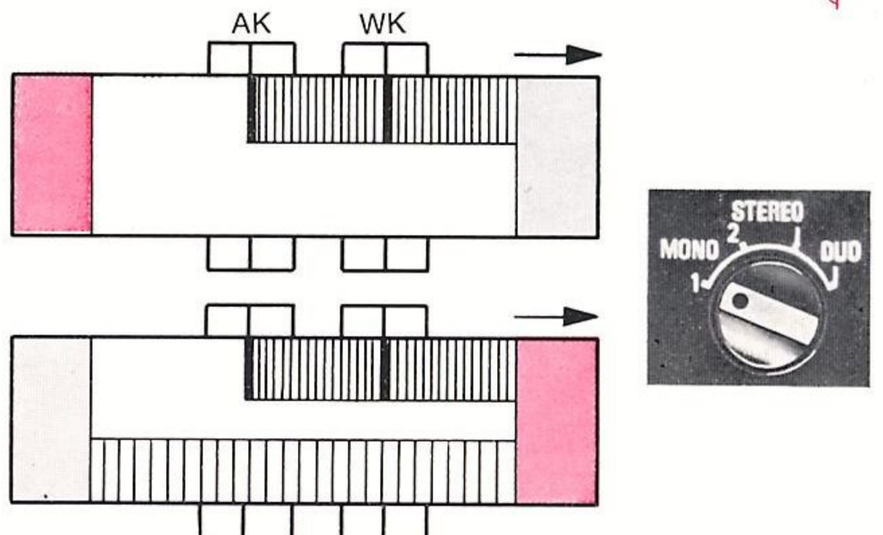
Skizze 6 Mono-Aufnahmen Halbspur
