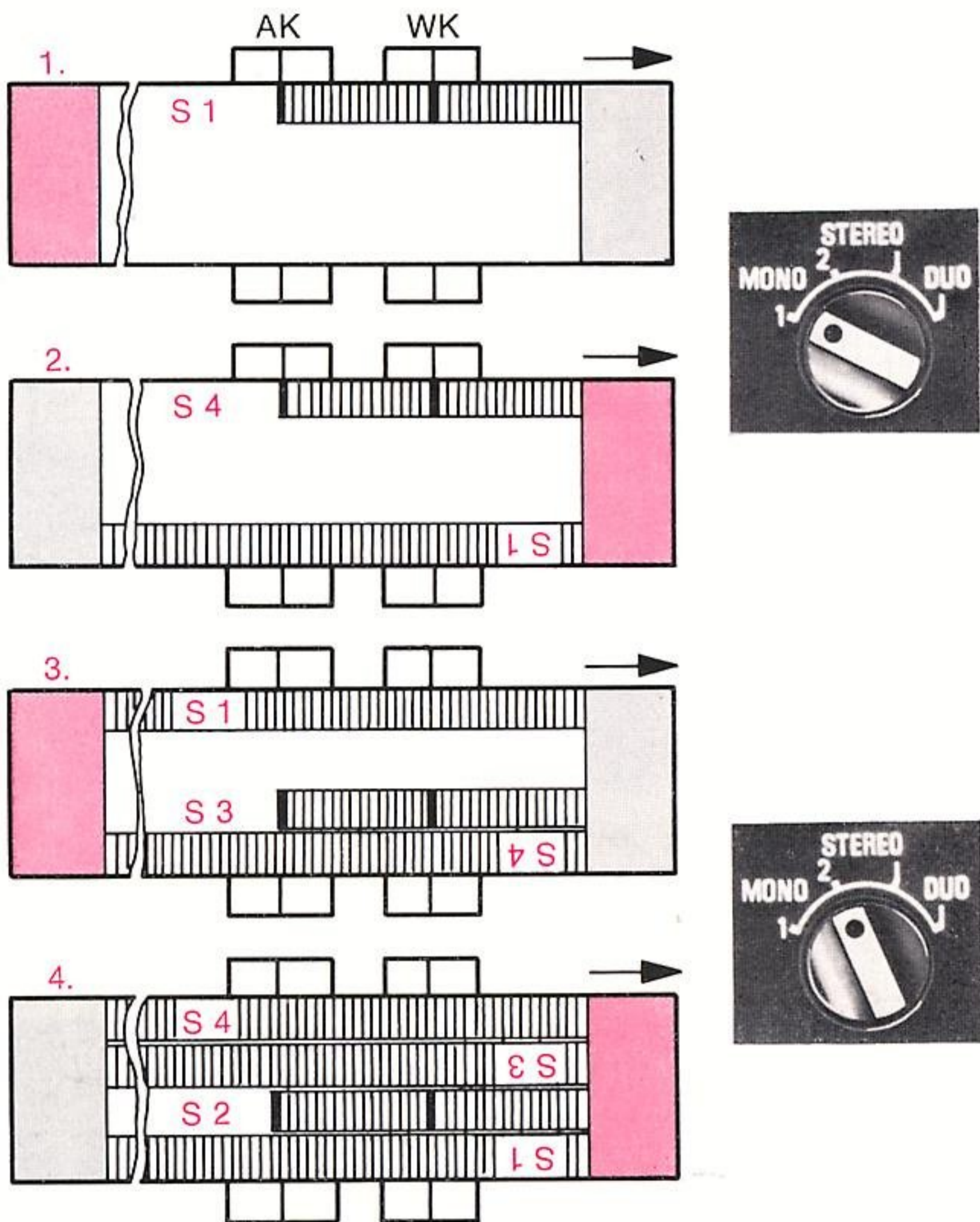
Skizze 2 Mono-Aufnahmen 4-Spur
