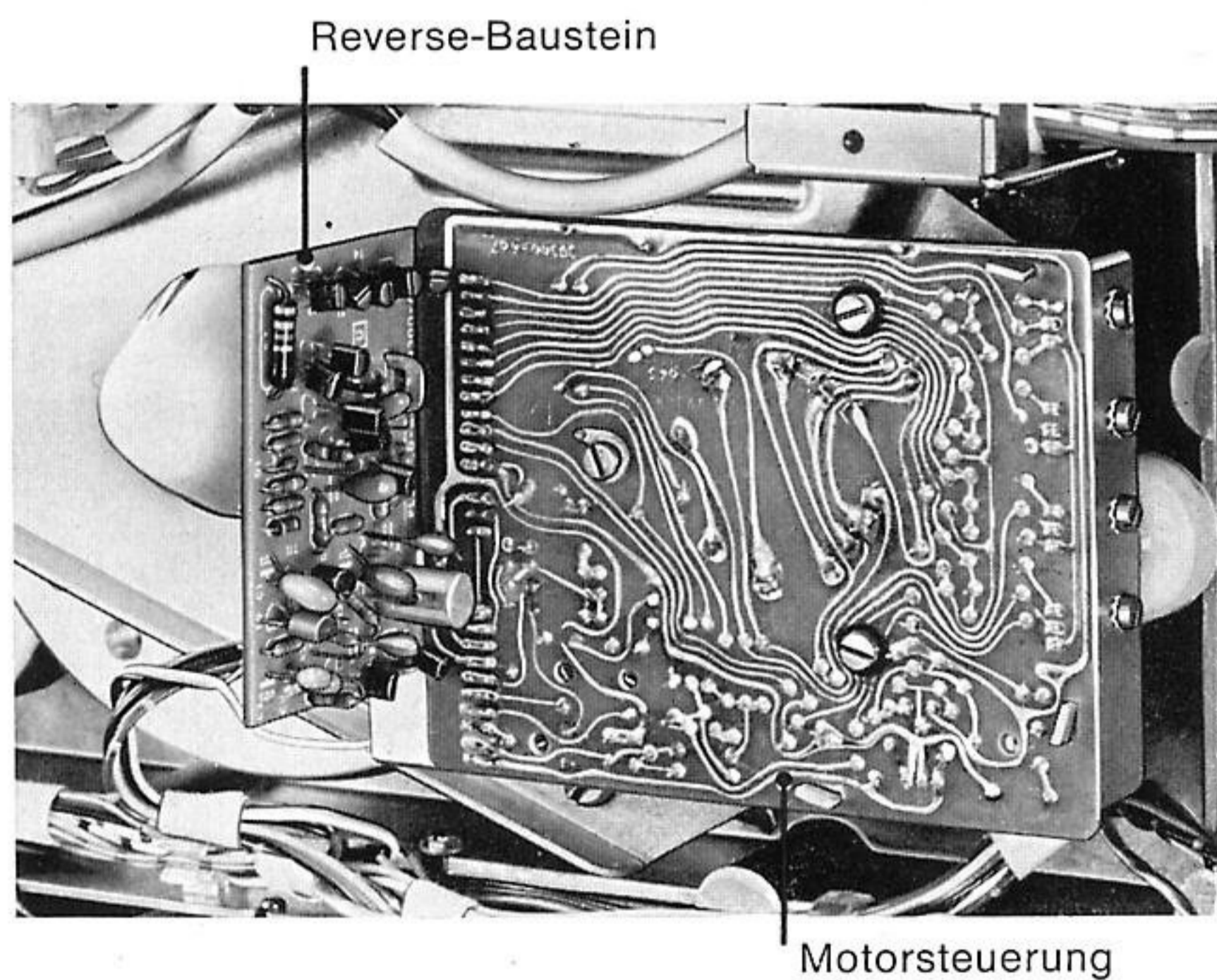
Reverse-Baustein einsetzen
