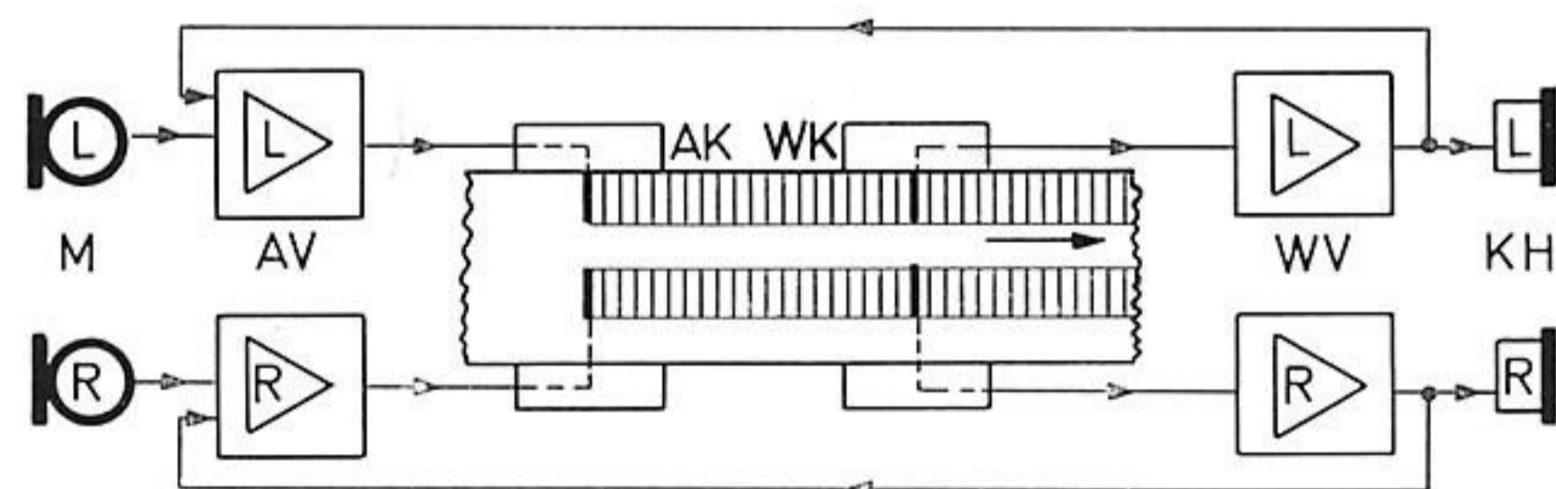
Echo-Aufnahme (Stereo)
