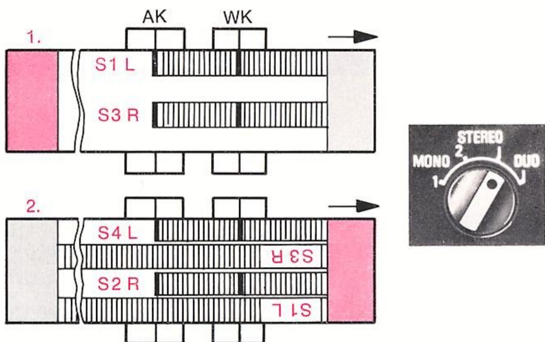
Skizze 3 Stereo-Aufnahme
