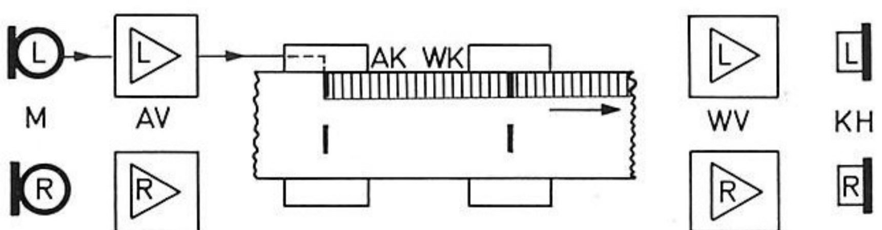
Multi-Playback 1. Aufnahme
